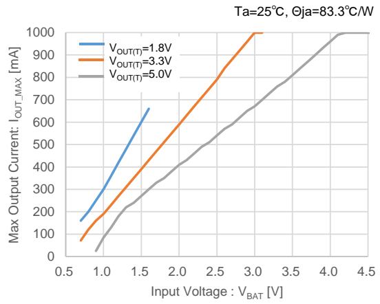
XC9147, f_{OSC}=3.0MHz
